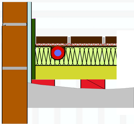
sol corrigé à l'aide d'un plancher en bois
