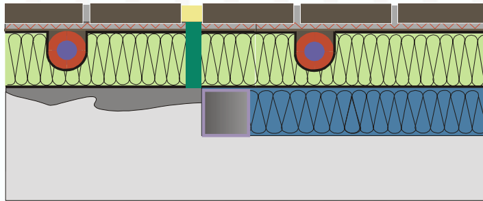
Égalisation de niveau avec panneau dur, support acier et joint de dilatation
