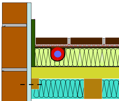
solution sans perte de hauteur
