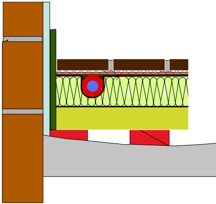
sol corrigé à l'aide d'un plancher en bois
