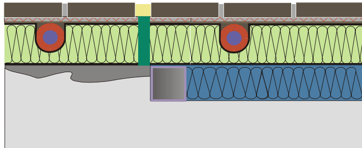
Égalisation de niveau avec panneau dur, support acier et joint de dilatation
