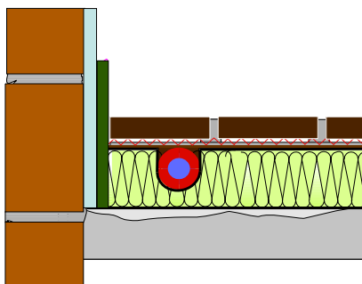
sol réparé et lisse
